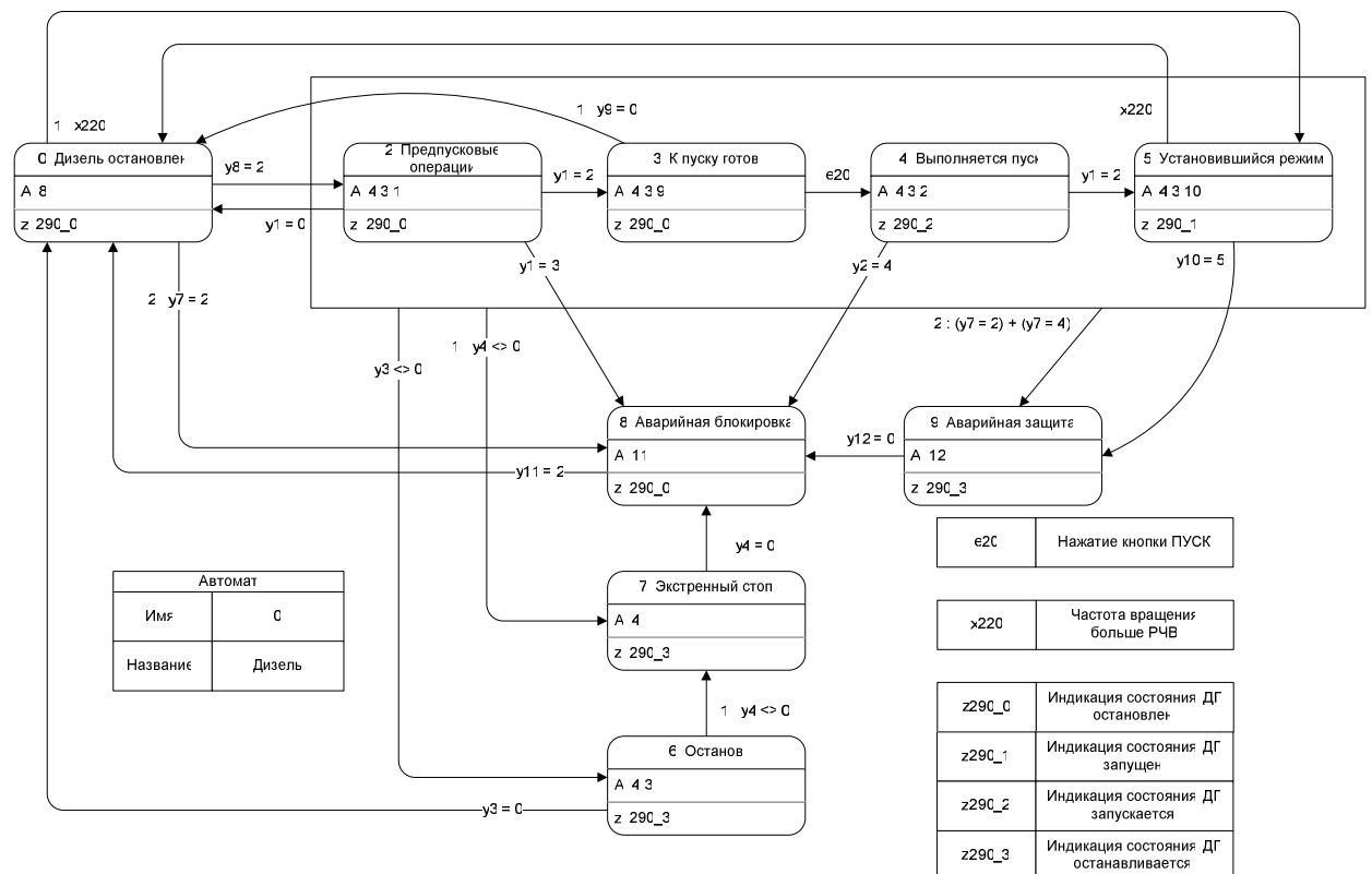
Рис. 2. Граф переходов автомата (страница A0 файла analizers.vsd )
