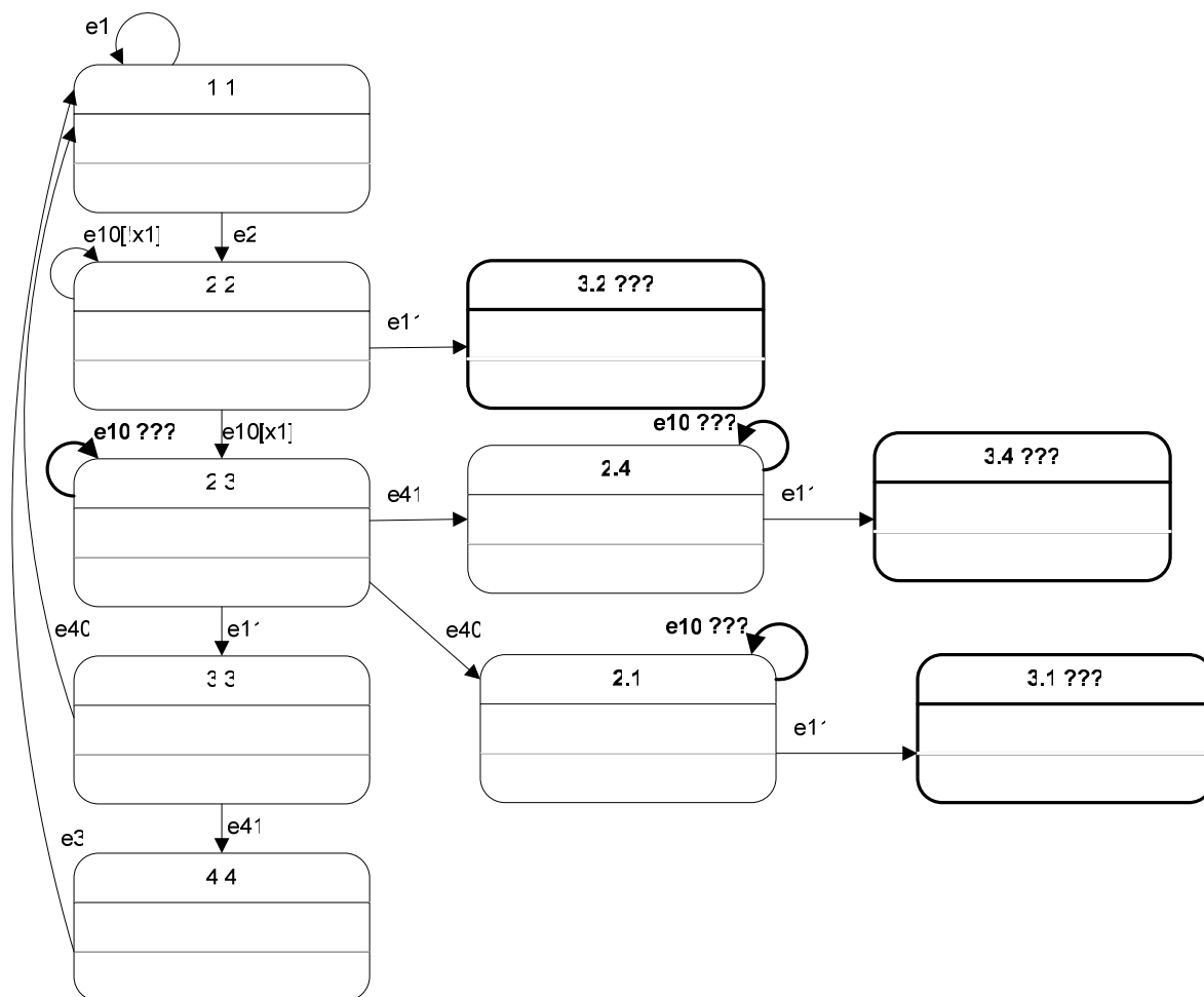
Рис. 4. Произведение автоматов «АТС» и «Телефон»
