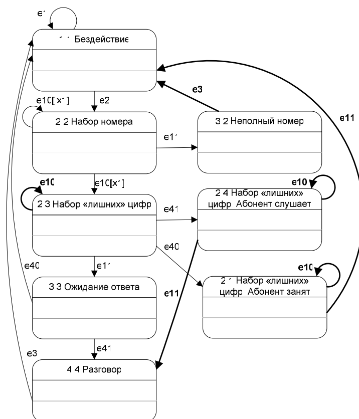
Рис. 5. Исправленное произведение автоматов «АТС» и «Телефон»
