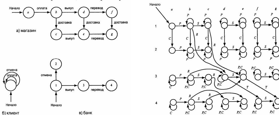
Рис. 2. Автоматы «Магазин», «Клиент» и «Банк» и их произведение из книги [2]
