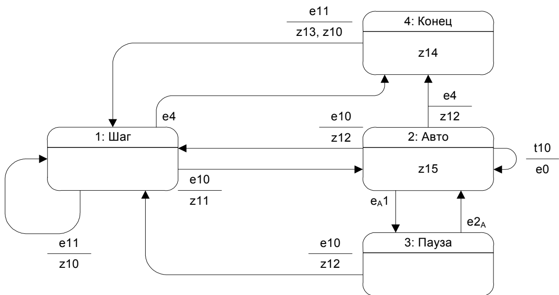
Рис. 14. Диаграмма переходов автомата интерфейса визуализатора
