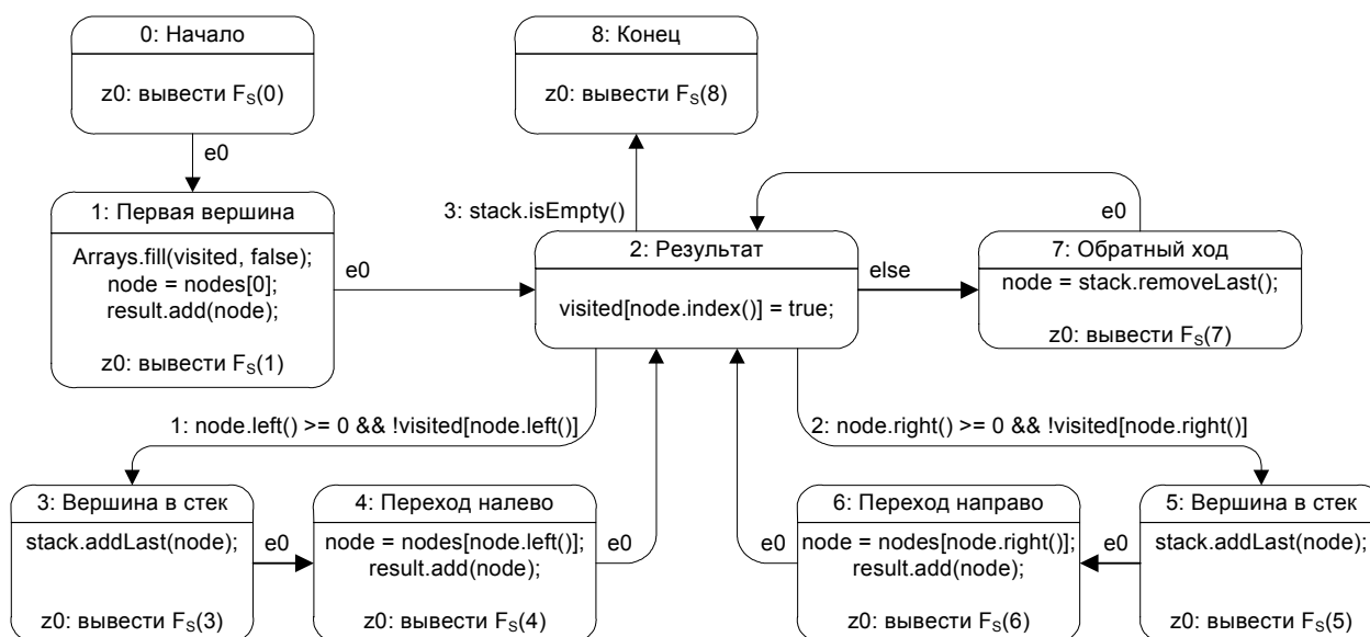
Рис. 7. Автомат визуализации
