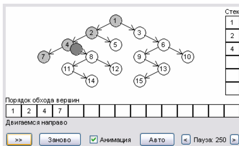
Рис. 12. Динамическая иллюстрация
