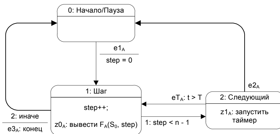
Рис. 3. Автомат анимации
