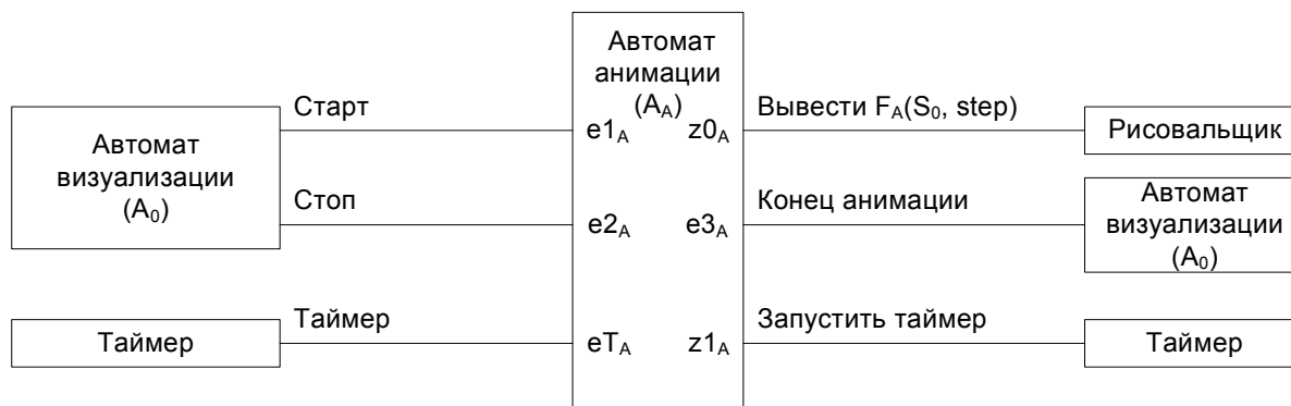
Рис. 4. Схема связей автомата анимации
