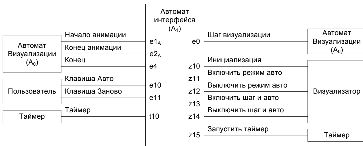
Рис. 13. Схема взаимодействия автомата интерфейса визуализатора
