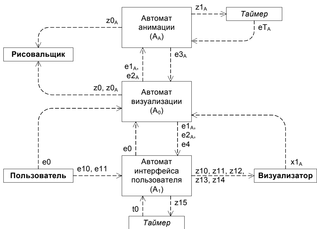
Рис. 16. Схема взаимодействия компонент визуализатора
