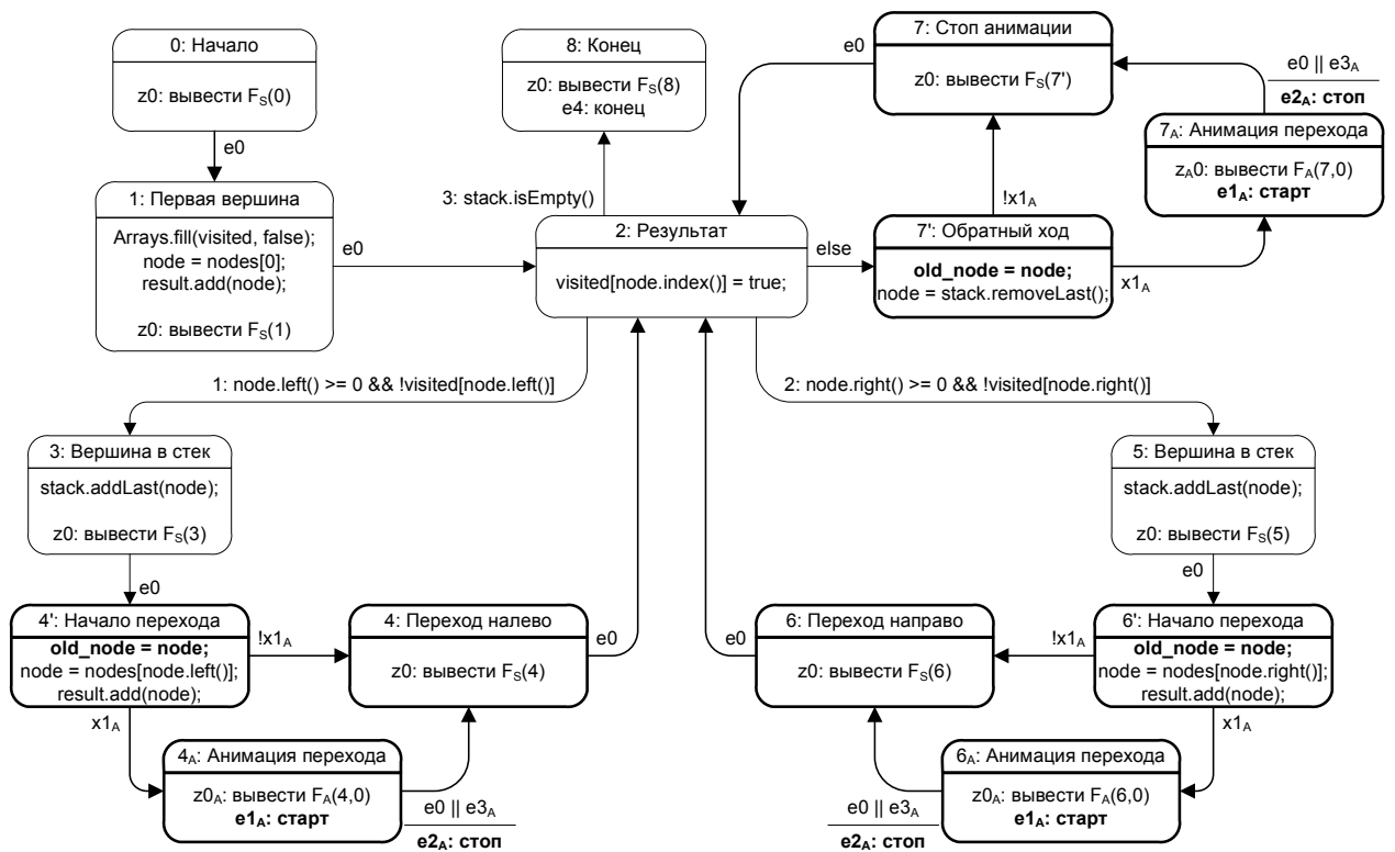
Рис. 8. Преобразованный автомат визуализации
