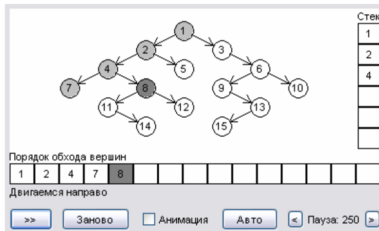
Рис. 9. Интерфейс визуализатора
