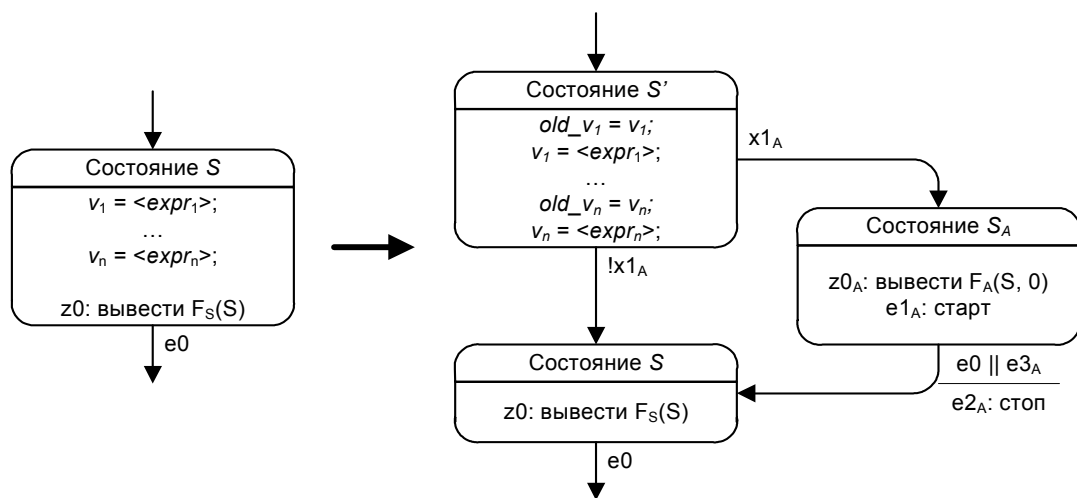
Рис. 2. Преобразование анимационного состояния
