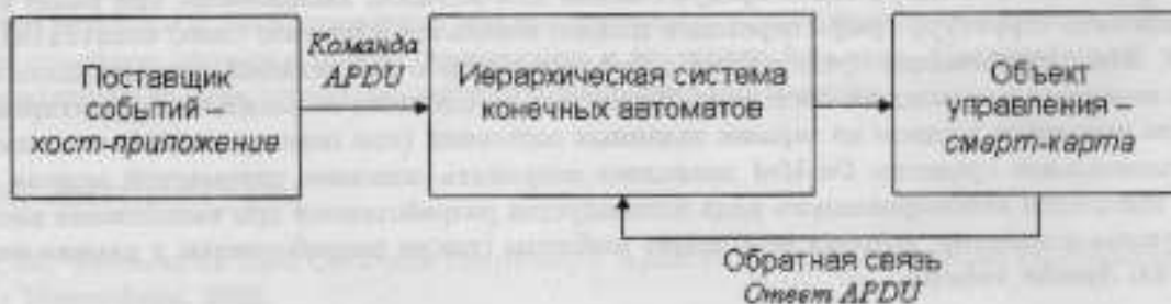
Рис. 2. Интерпретация автоматного программирования для платформы Java Card
