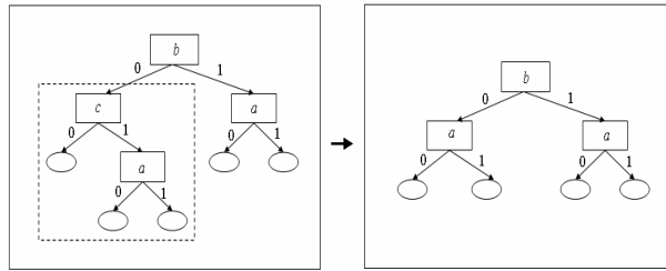
Рис. 2. Мутация деревьев решений
