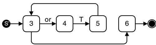
■ Рис. 4. Удаление правой рекурсии на диаграмме состояний для нетерминала S'
