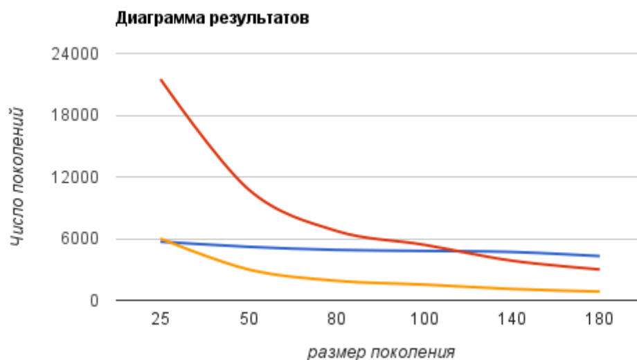
Рис 1. Первые результаты измерений Красный — OpenCL (CPU), синий — OpenCL (GPU), желтый — CPU (5 потоков)
