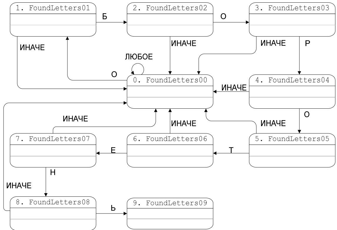
Рис. 3. Недетерминированный автомат для поиска слова оборотень
