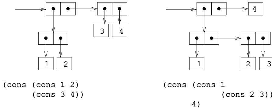
Рис. 2.3: Два способа соединить 1, 2, 3 и 4 с помощью пар.
