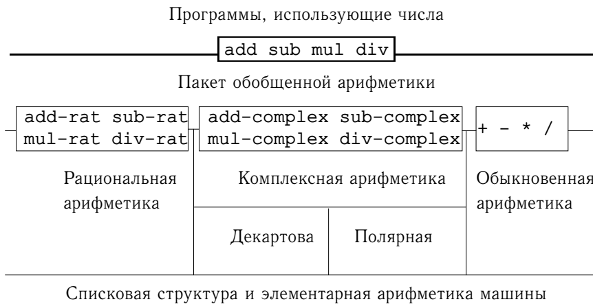
Рис. 2.23: Обобщенная арифметическая иерархия.
