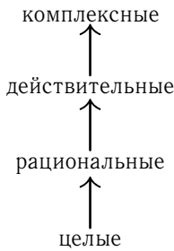
Рис. 2.25: Башня типов
