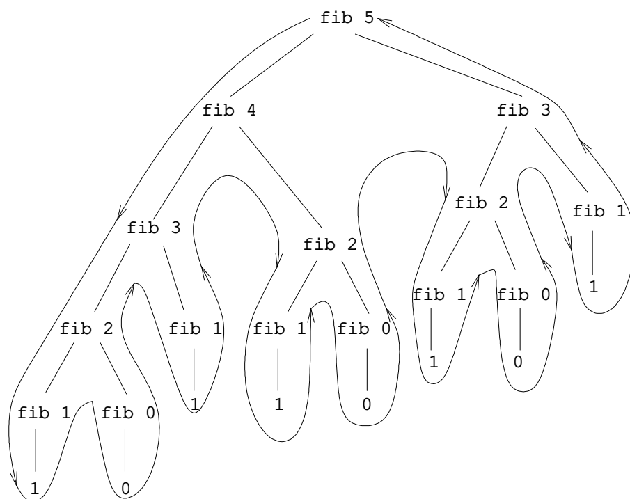
Рис. 1.5: Древоподобно-рекурсивный процесс, порождаемый при вычислении (fib 5).
