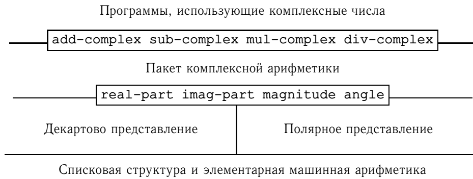
Рис. 2.21: Структура обобщенной системы комплексной арифметики.
