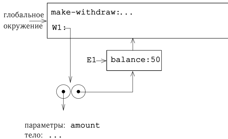
Рис. 3.9: Окружения после вызова W1.
