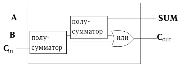
Рис. 3.26: Сумматор.
