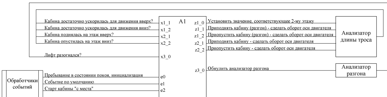
Рис. 3. Схема связей автомата A1.
