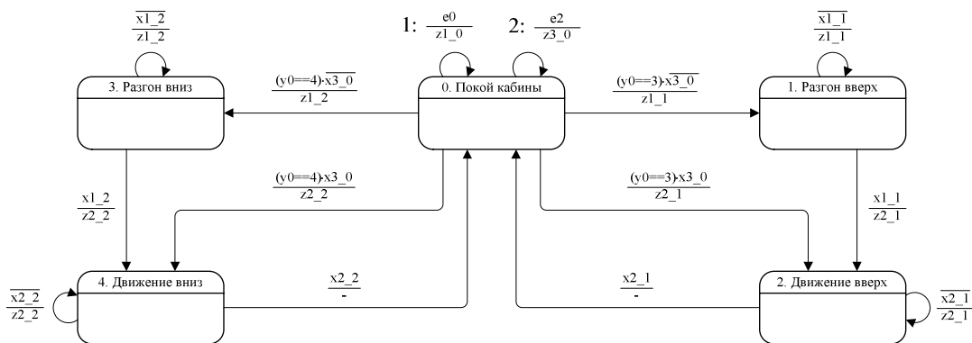
Рис. 4. Граф переходов автомата A1.
