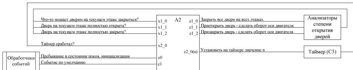
Рис. 5. Схема связей автомата A2 .
