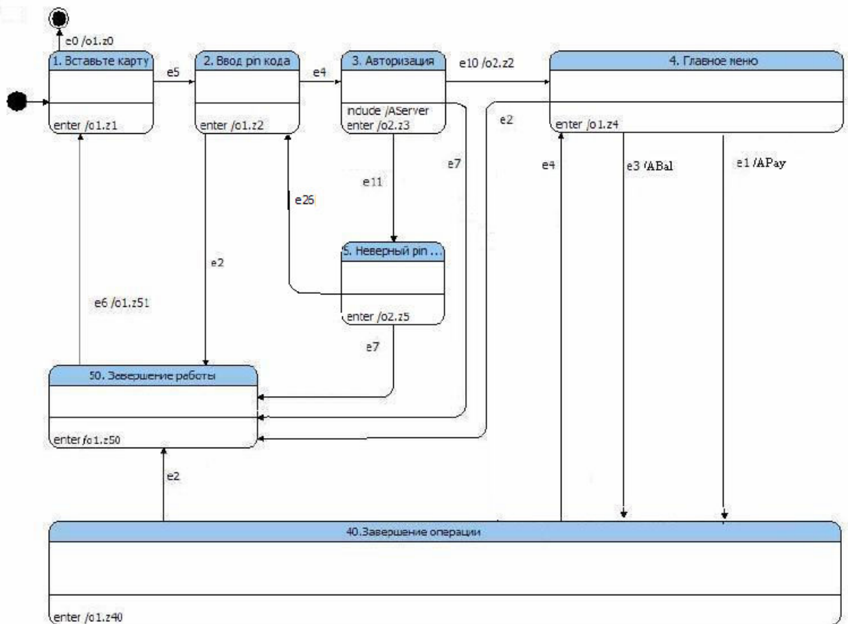
Рис. 17. Граф переходов автомата, отвечающего за работу банкомата
