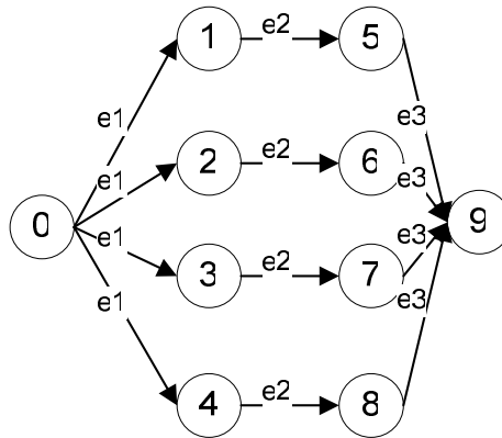
Рис. 6. Граф переходов до слияния состояний
