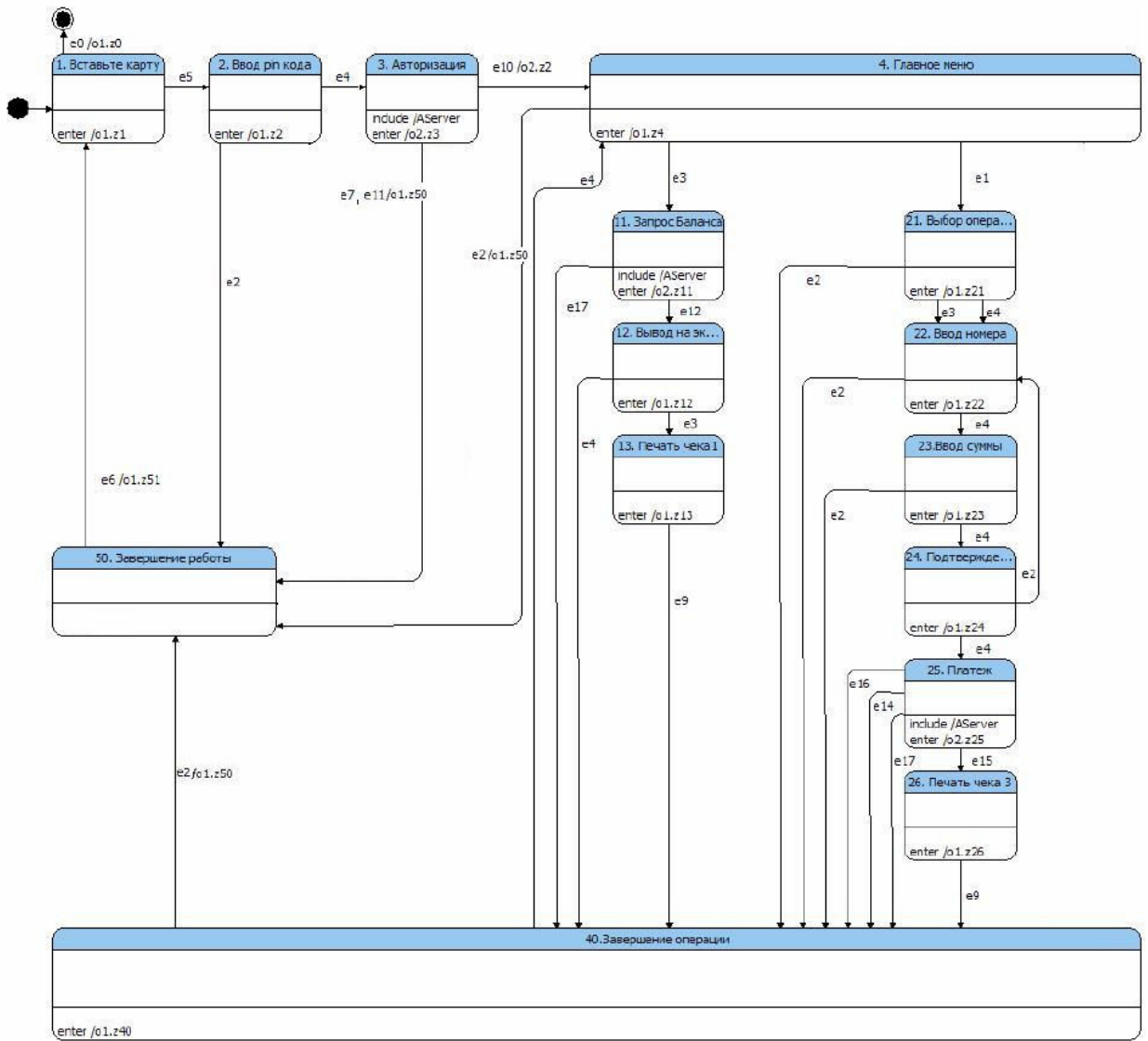
Рис. 13. Граф переходов автомата, отвечающего за работу банкомата
