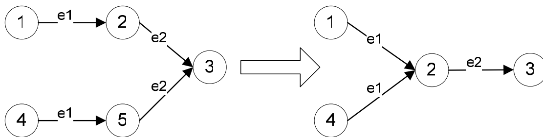
Рис. 5. Слияние состояний
