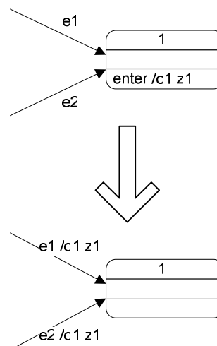
Рис. 10. Перемещение воздействия из состояния в переходы
