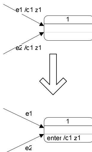
Рис. 11. Перемещение воздействия из переходов в состояние
