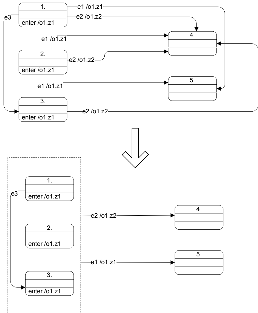
Рис. 1. Группировка состояний
