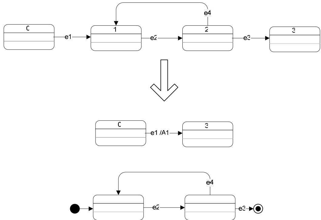
Рис. 8. Выделение автомата
