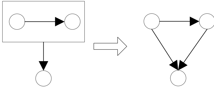
Рис. 4. Удаление группы состояний
